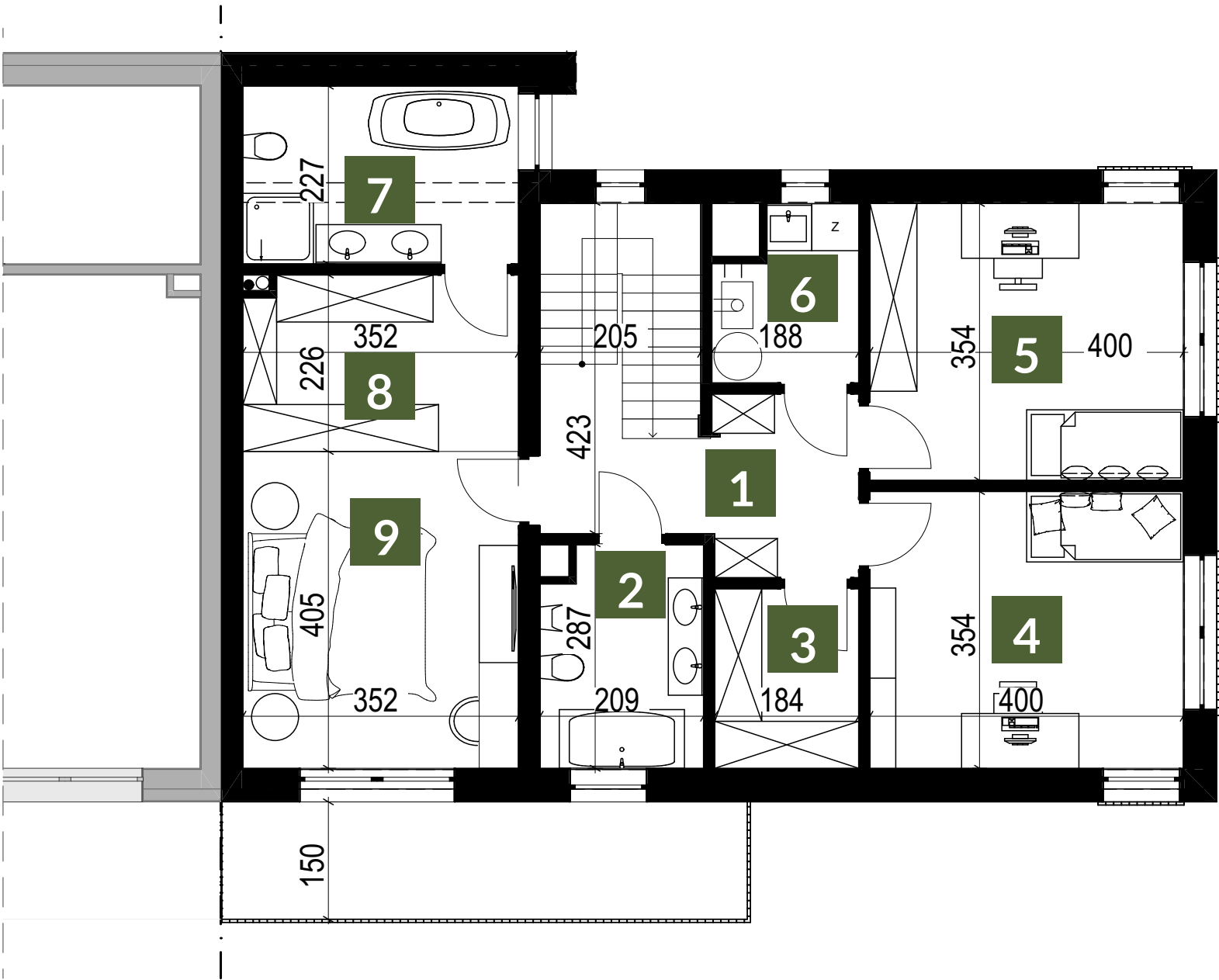
RZUT PODDASZA
