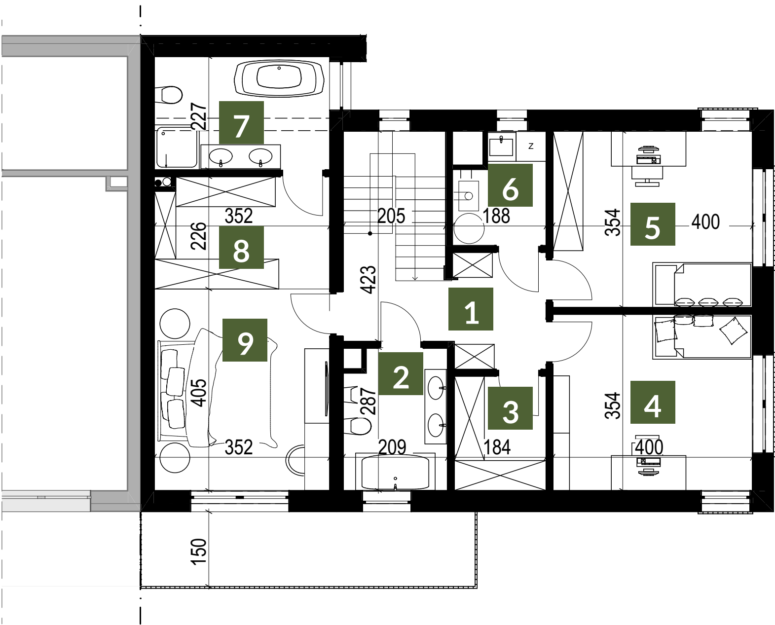
RZUT PODDASZA
